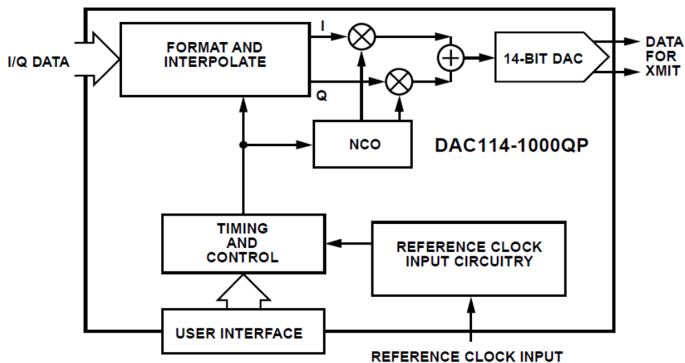
图1、DAC114-1000QP功能框图
