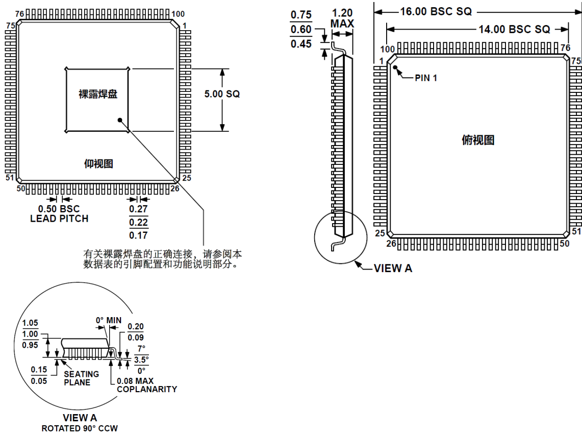
100 引脚裸露焊盘、超薄四方扁平封装[TQFP_EP](SV-100-4)尺寸(单位:mm)
